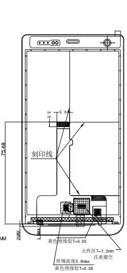
FPC弯折示意图 FPC弯折出货
